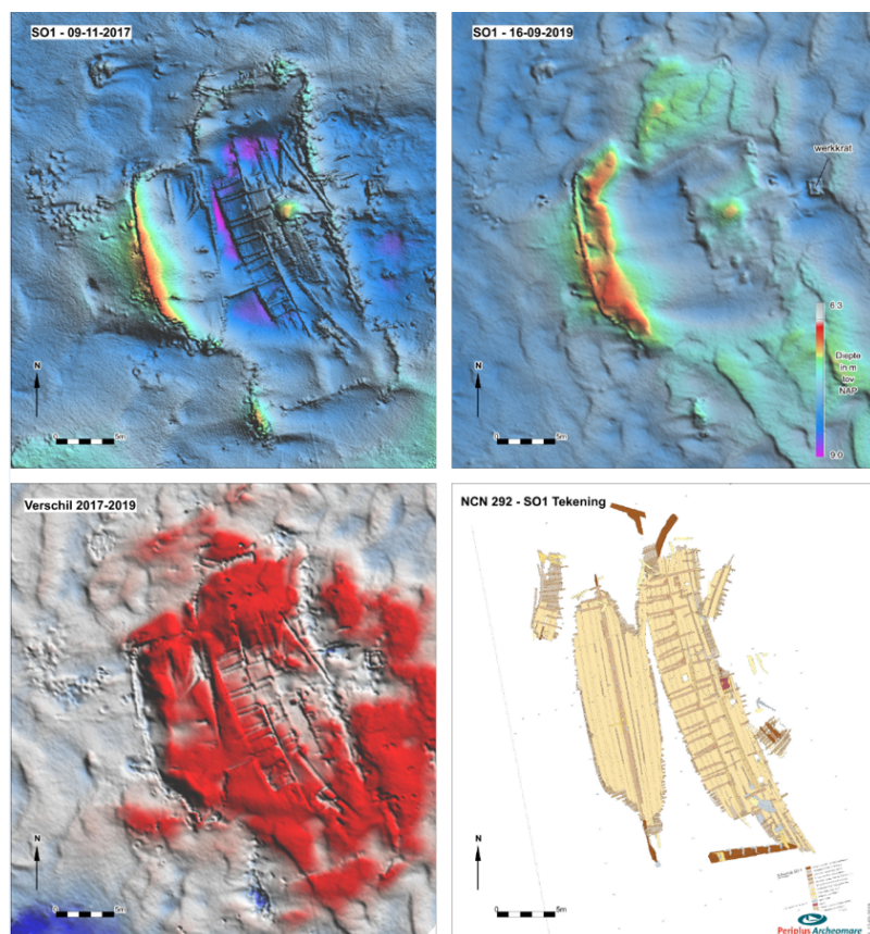
Multibeam opname van het scheepswrak Scheurrak SO1. Door het aanbrengen van steigergaas netten ligt de houten constructie weer onder een beschermende laag sediment (Afbeelding: Periplus Archeomare).
